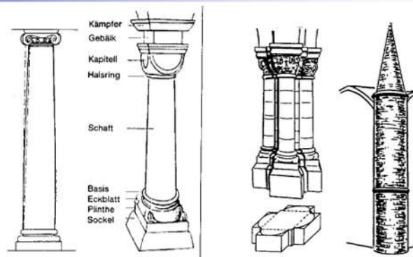
Säule Pfeiler
