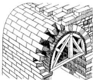
Tonnengewölbe
